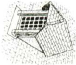
lucarne à demi-croupe, dite normande
